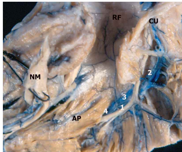
Fig. 13. 1, Ramo profundo del nervio ulnar (RPNU); 2, Rama palmar profunda de la arteria ulnar, disposición proximal (PRPAU); 3, continuación rama palmar profunda de la arteria ulnar (RPAU); 4, Arteria radial (AR); CU, Canal ulnar; RF, Retináculo flexor del carpo; AP, Aductor pollicis; NM, Nervio mediano.
